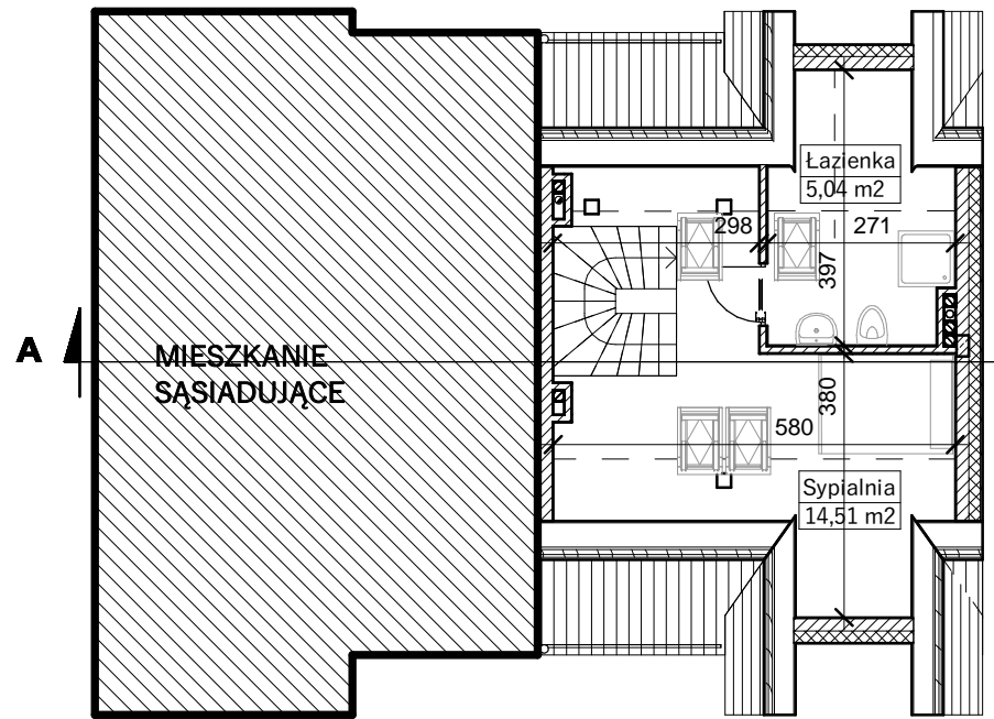
RZUT PODDASZA
