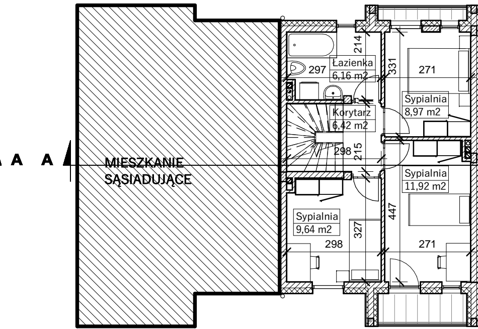
RZUT PIĘTRA
