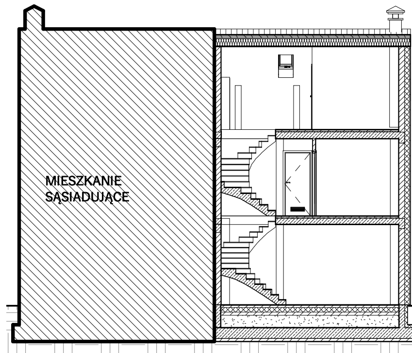
PRZEKRÓJ A - A
