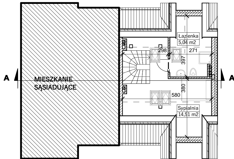
RZUT PODDASZA
