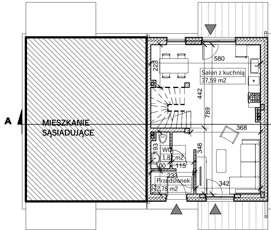
RZUT PARTERU
