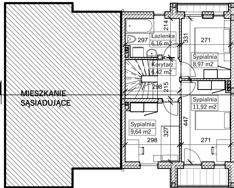
RZUT PIĘTRA
