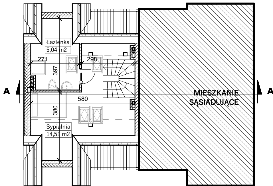
RZUT PODDASZA
