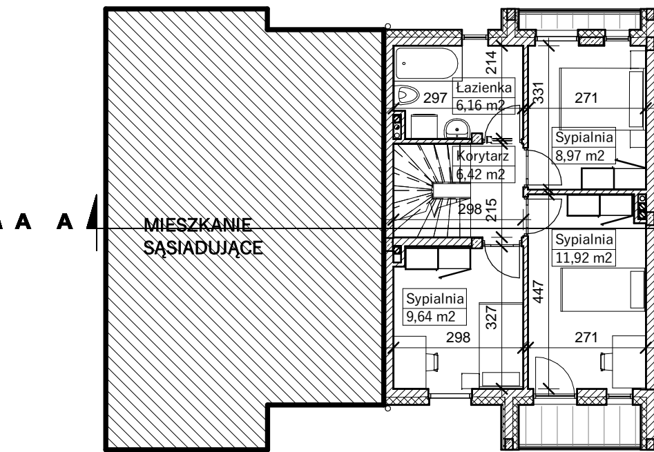
RZUT PIĘTRA
