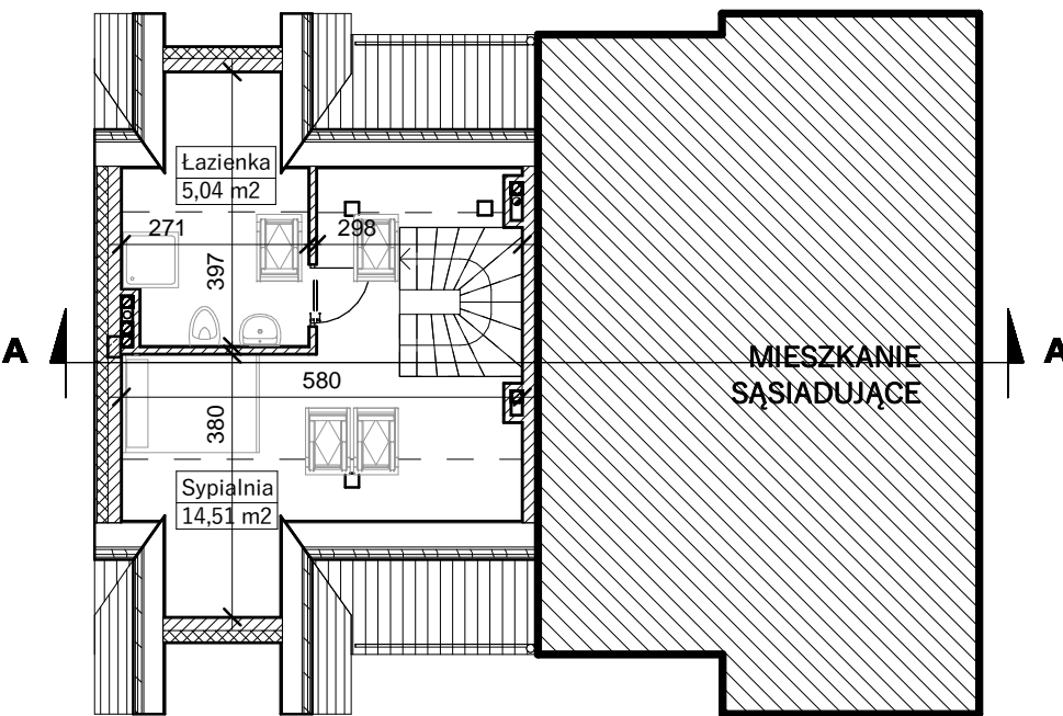
RZUT PODDASZA
