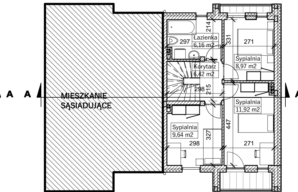
RZUT PIĘTRA
