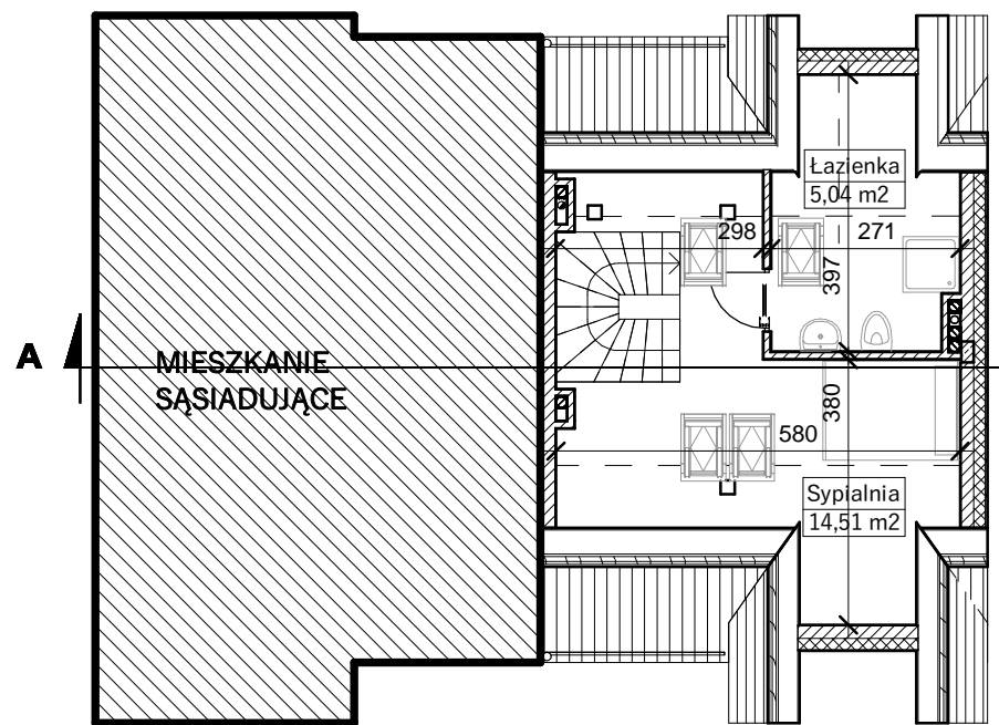
RZUT PODDASZA
