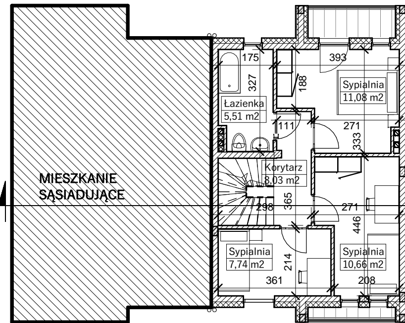
RZUT PIĘTRA
